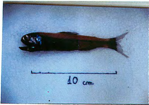
Diaphus adenomus
