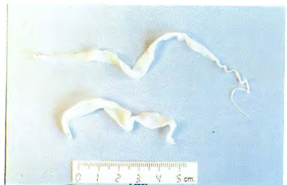
Leptocephali
