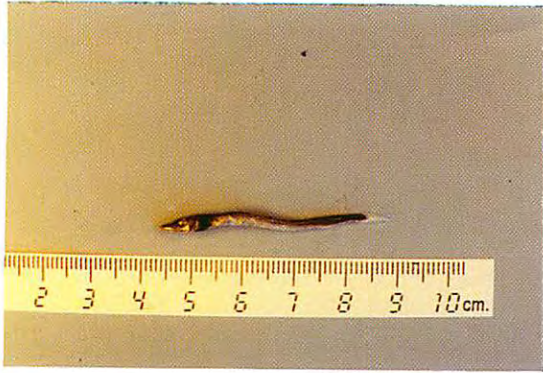
Scopelosaurus argenteus
